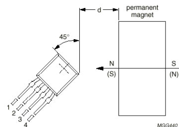
Detector de Proximidad utilizando un sensor magneto-resistivo.
