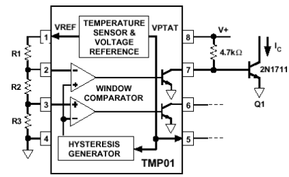
Salida con transistor
