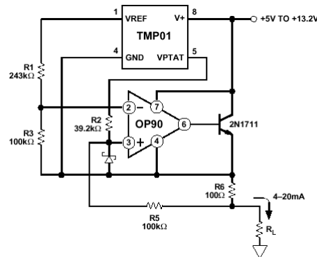
Salida con lazo de corriente 4-20mA
